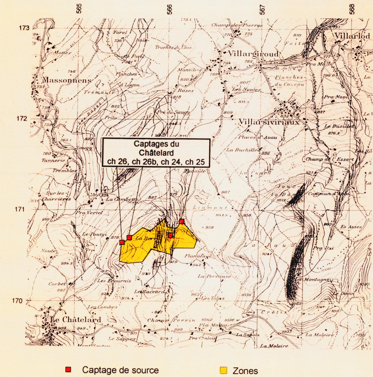
Plan de situation (Extrait de la C. N. 1 : 25'000, Feuille 1204, Romont et 1224, Moudon)
